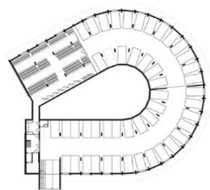
Halfverdiepte kelder
