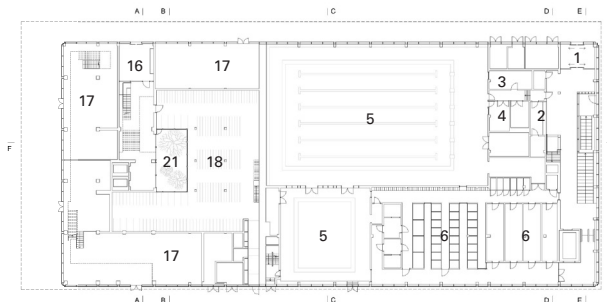
plattegrond 00
