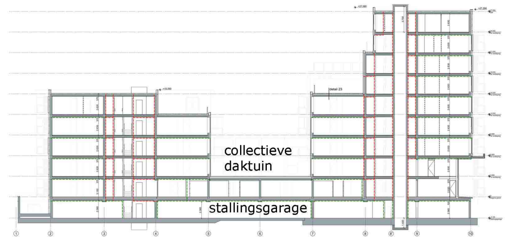
doorsnede west-oost
