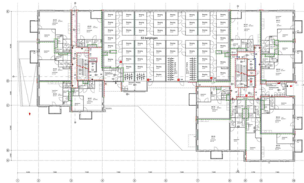
Begane grond
