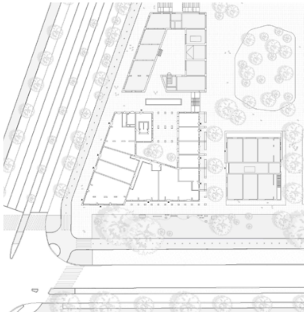
Situatietekening MO*town Track 8
