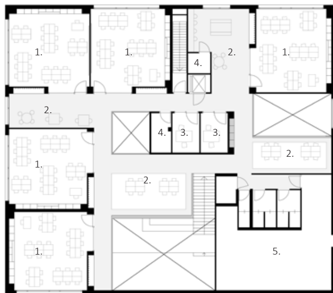
Plattegrond eerste verdieping
