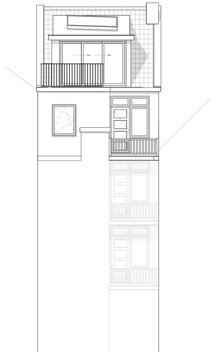
achtergevel
